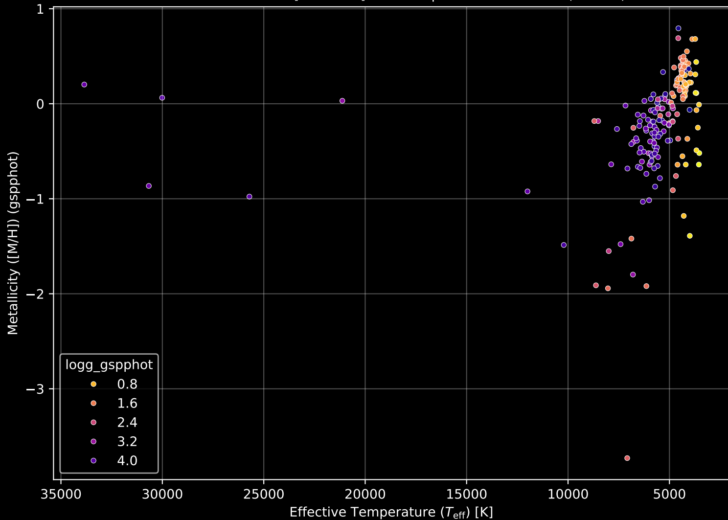
APOGEE DR17 Field: [281-36-O] Stellar Population Parameters (n= 188)
