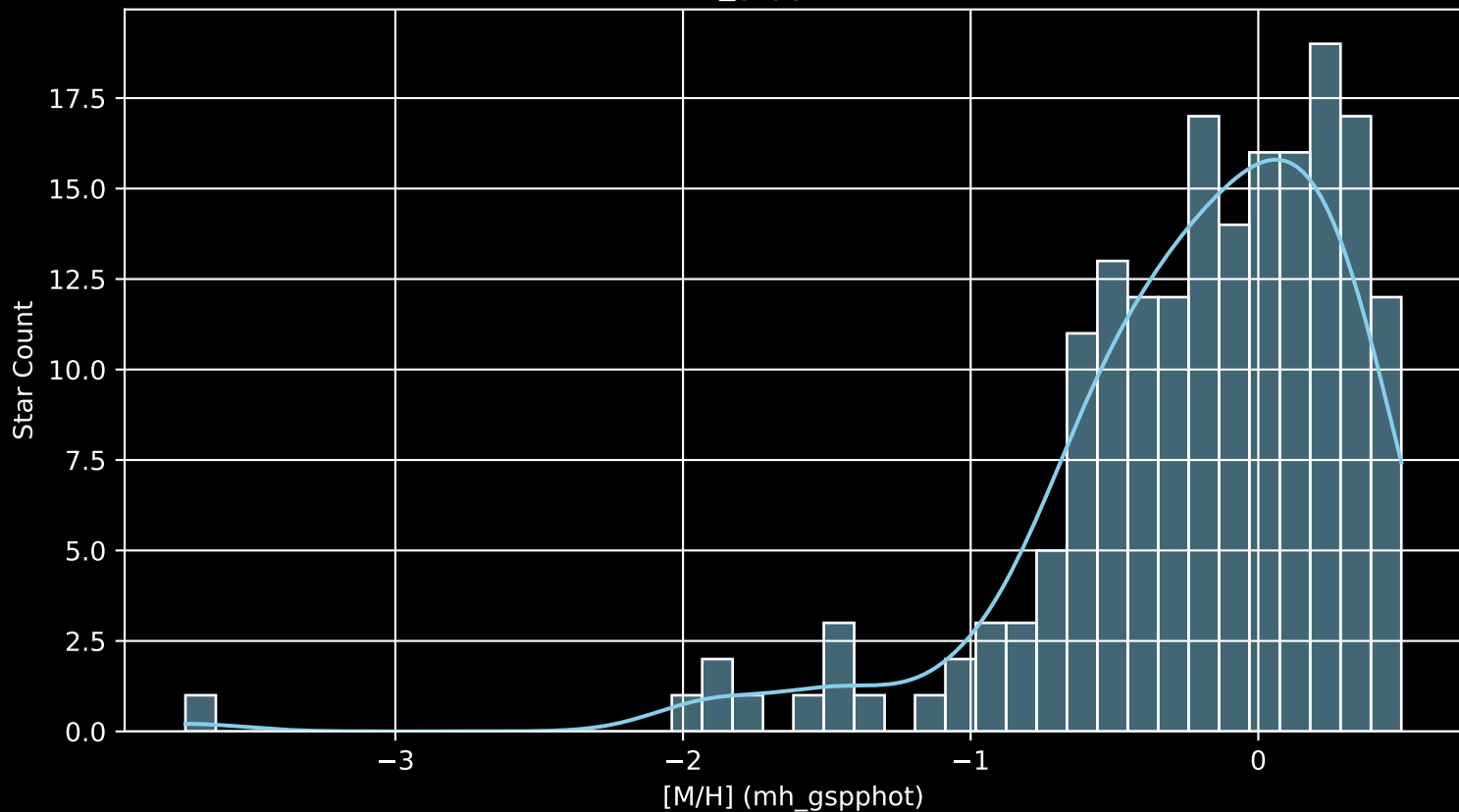
APOGEE DR17 Field: [281-36-O [M/H] (mh_gspphot) (n= 183)
